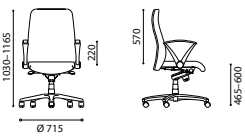
Indiana mit höhenverstellbaren Armlehnen und verchromtem Fußkreuz aus Stahl
